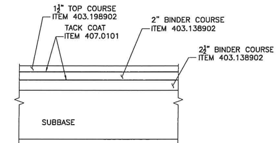
RECONSTRUCTION PAVEMENT SCALE: N.T.S.
