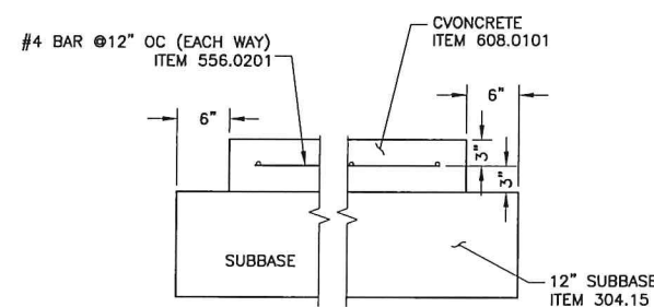
CONCRETE PAD DETAIL SCALE: N.T.S.
