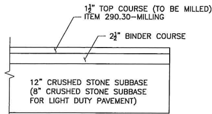
EXISTING PAVEMENT SCALE: N.T.S.
