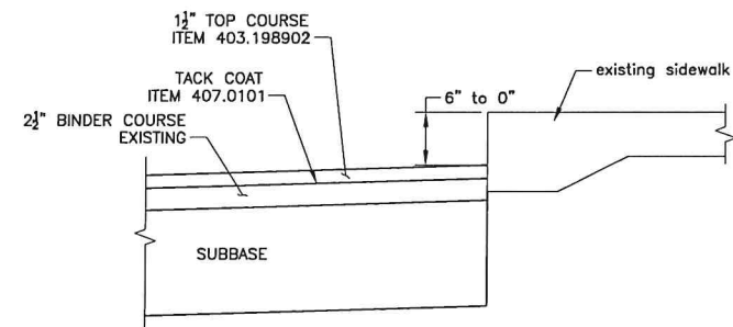
TYPICAL CURB SECTION SCALE: N.T.S.
