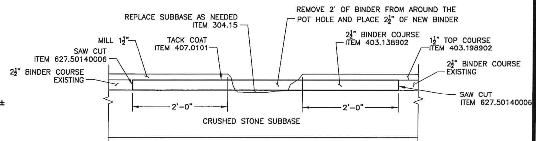
SECTION VIEW POT HOLE REPAIR SCALE: N.T.S.
